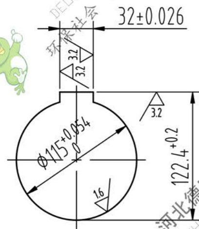
轴孔图
